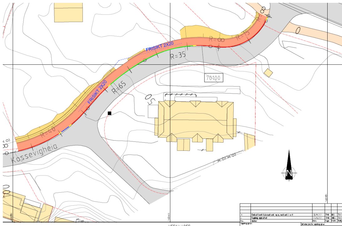
Figur 3. Teknisk plan for fortau i reguleringsplan 201218, C-tegning.
