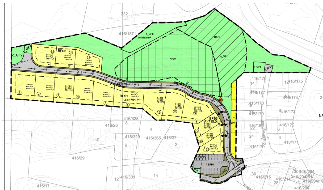
Figur 1 Reguleringsplan for Kossevigheia nord – planid 1518, vedtatt 09.06.2021.
