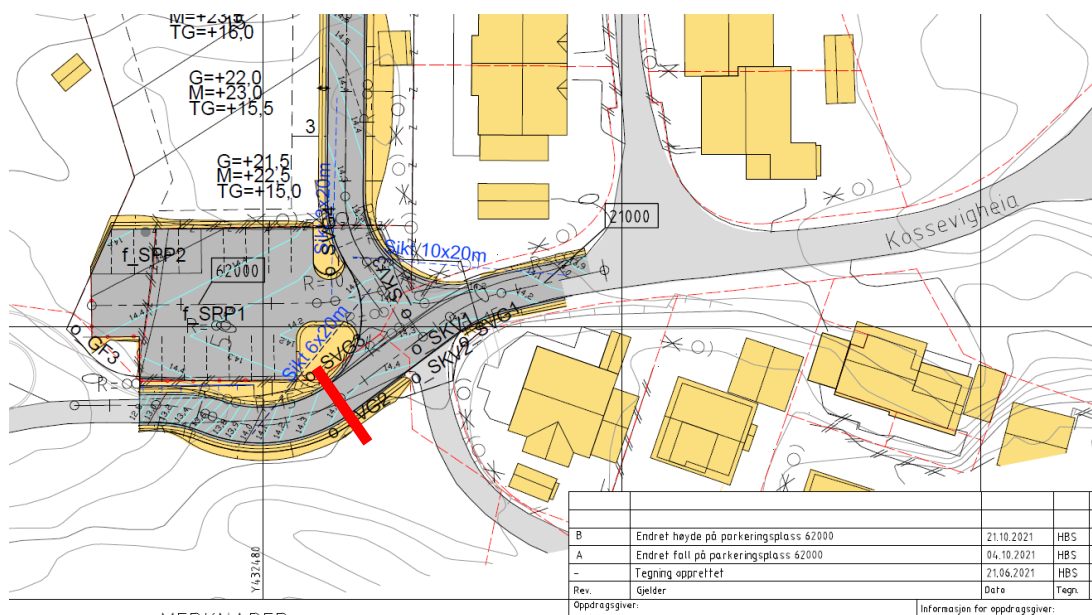
Figur 4. Utsnitt av teknisk plan for vei i reguleringsplan 1518, C-tegning. Del av eksisterende vei Kossevigheia skal utbedres til og med krysset inn til Kossevigheia nord (grense markert med tykk rød strek)
